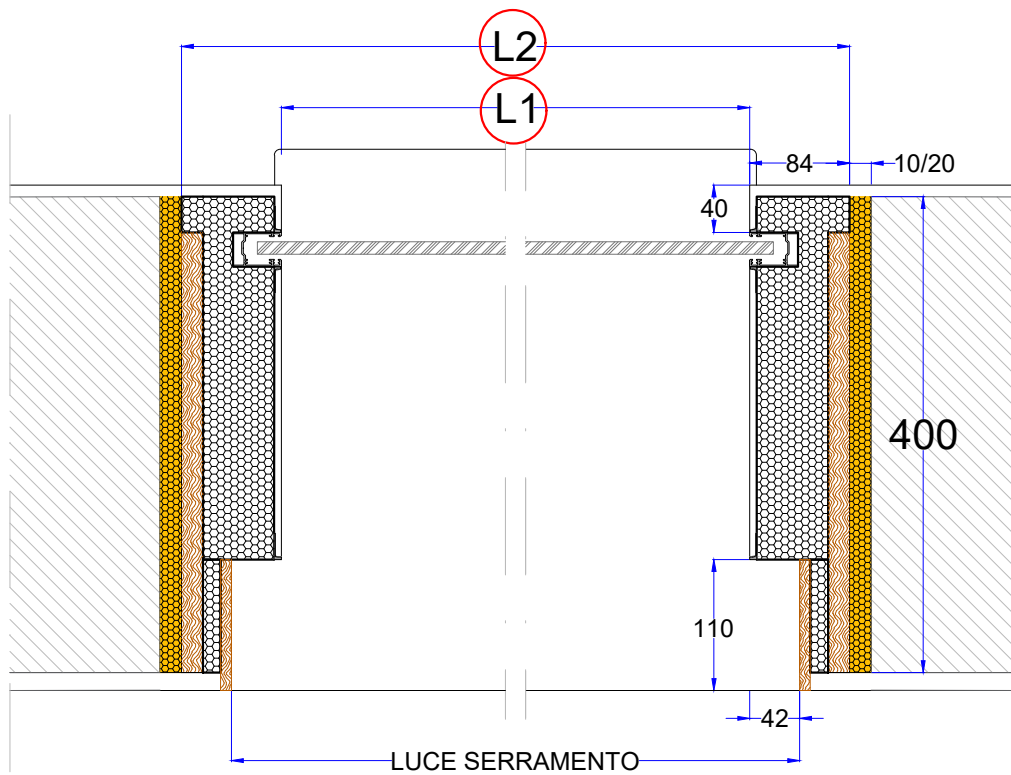
S e z i o n e O r i z z o n t a l e
